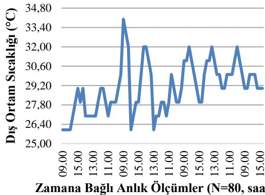
Şekil 5. Hava kaynaklı ısı pompasının bulunduğu bölgedeki dış ortam sıcaklık değerleri (Outdoor temperature values in the area where the air source heat pump is located)
