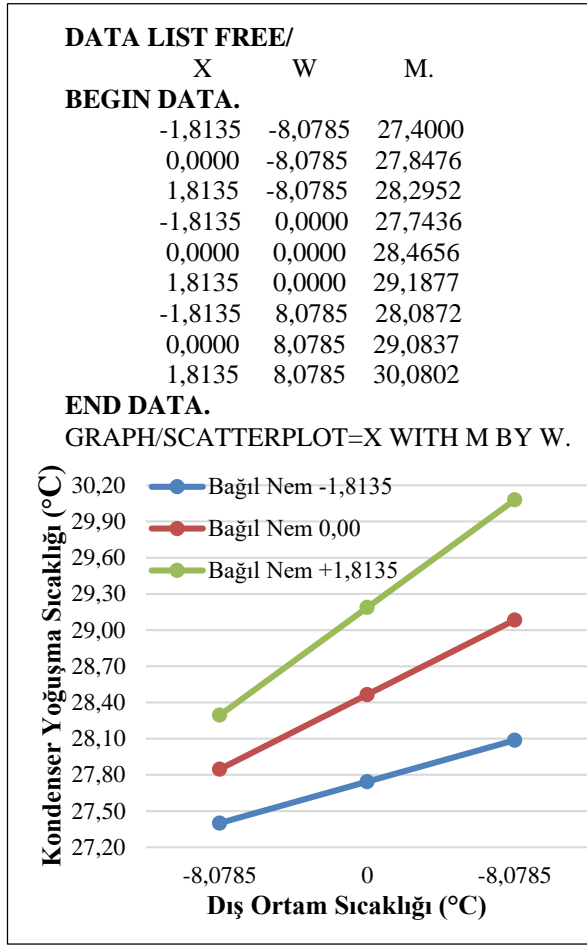
Şekil 11. Bağıl nem, dış ortam sıcaklığı ve kondenser yoğuşma sıcaklığı arasındaki etkileşimlere ait grafik (Graph of the interactions between relative humidity, outdoor temperature and condenser condensation temperature)
