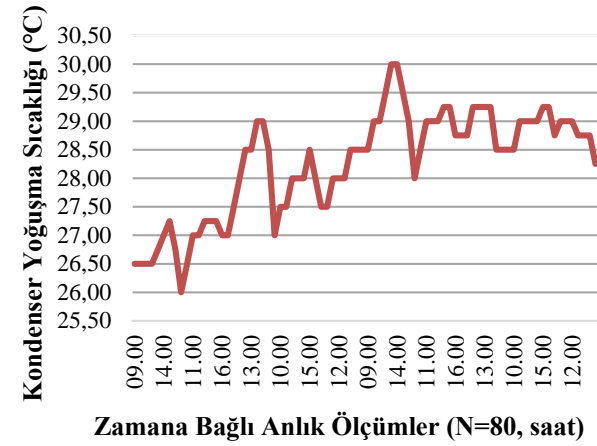
Şekil 2. Kondenser yoğuşma sıcaklığı ölçümleri (Condenser condensation temperature measurements)
