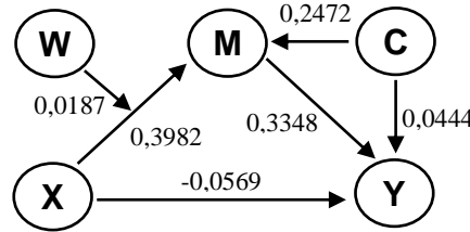
Şekil. Optimizasyon modelin kavramsal diyagramı. / Figure. Conceptual diagram of the optimization model.
