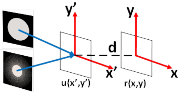
Figure 8. Optical propagation geometry for the aperture functions ( A_{AMDL} , A_{MDL} ) (Açıklık fonksiyonları için optik yayılma geometrisi ( A_{AMDL} , A_{MDL} ))
