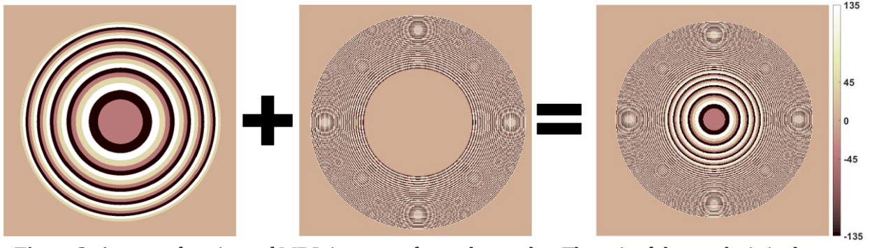
Figure 3. Aperture functions of MDL in terms of complex angles. The unit of the graphs is in degrees. (Karmaşık açılar cinsinden MDL'nin açıklık fonksiyonları. Grafiklerin birimi derecedir.)
