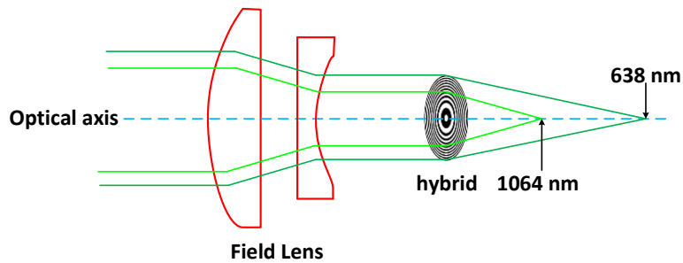
Figure 11. Illustration of an electro-optic system using the two-foci diffractive lens system (iki odaklı kırınımlı mercek sistemi kullanan bir elektro-optik sistemin gösterimi)
