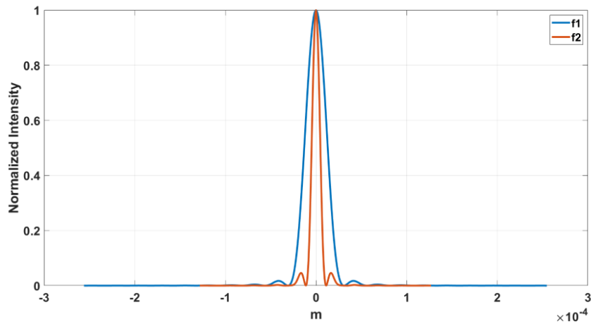
b) Cross section of normalized intensity distributions of the AMDL (AMDL'nin normalizeştirilmiş şiddet dağılımlarının kesiti.)
