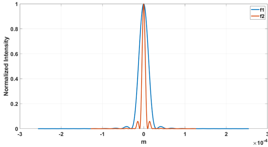
a) Cross section of normalized intensity distributions of the MDL (MDL'nin normalizeştirilmiş şiddet dağılımlarının kesiti.)
