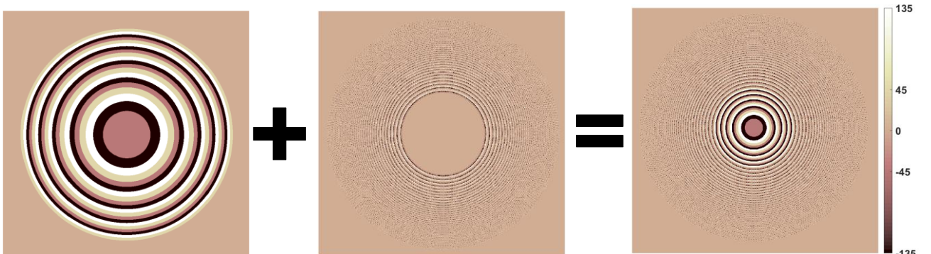
Figure 4. Aperture function of AMDL in terms of complex angles. (Kompleks açılar cinsinden AMDL'nin açıklık fonksiyonu.)
