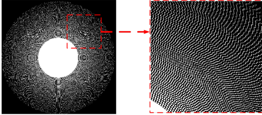
a) Aperture function of the AMDL in terms of magnitude. (AMDL'nin açıklık fonksiyonu büyüklük cinsinden)
