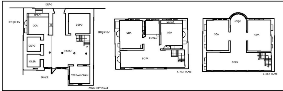
Şekil 5. Ali Osman Tosun Evi kat planları (Sayan, 1995 çizimlerinden güncellenmiştir) (Ali Osman Tosun House floor plans (updated from Sayan, 1995 drawings))
