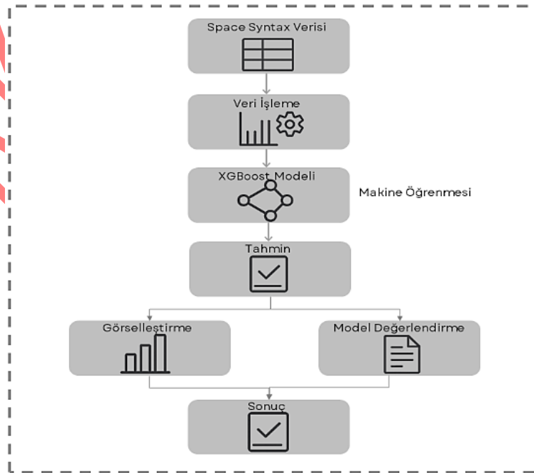
Şekil 4. Yöntem akış şeması (Method flowchart)
