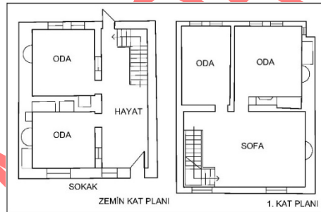
Şekil 11. İsmail Göker Evi kat planları (Sayan, 1995 çizimlerinden güncellenmiştir) (İsmail Goker House floor plans (updated from Sayan, 1995 drawings))
