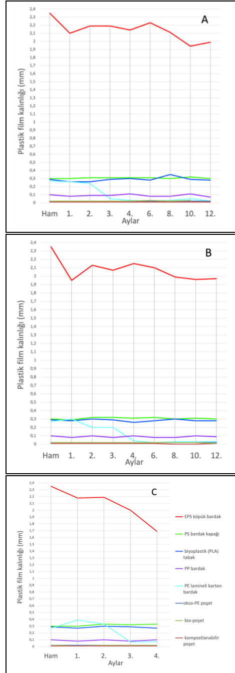
Şekil 6. Numunelerin kalınlıkları değişimi, deniz (A): Toprak (B): ve göl (C).
