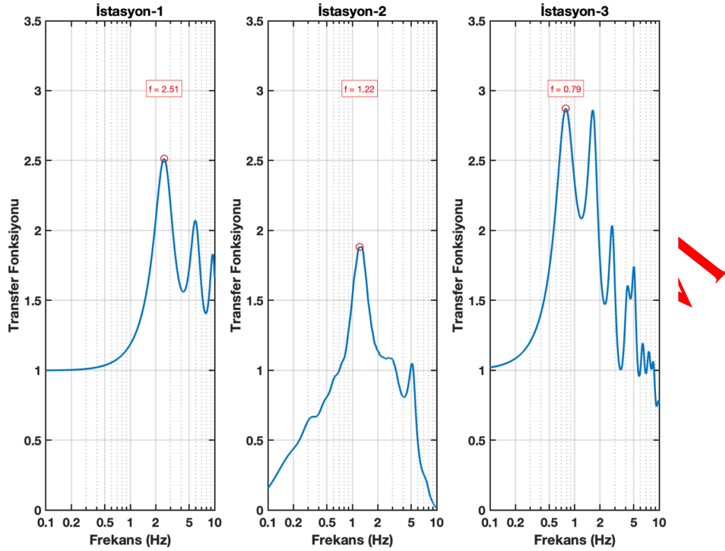
Şekil 4. İvme istasyonlarında hesaplanan transfer fonksiyonları ve hakim frekans değerleri (The transfer functions and dominant frequencies calculated at the acceleration stations)
