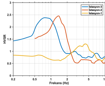
Şekil A: Her istasyon için mikrotremor ölçümlerinden elde edilmiş HVSR eğrileri / Figure A: The HVSR curves obtained from microtremor measurements for each station
