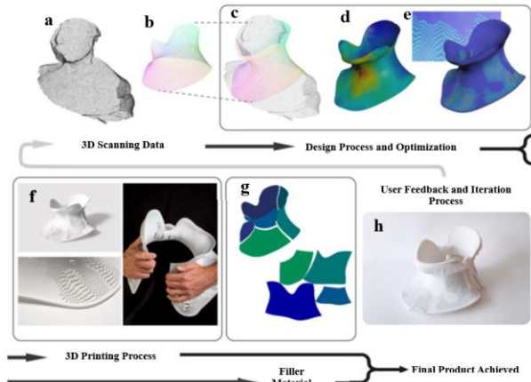
Figure 6. Manufacturing process of a custom-designed orthosis using 3D printing: a) 3D scanning, b) and c) designed orthosis, d) and e) design optimization, f) 3D-printed orthosis, g) orthosis infill trimming through variable surface cutting algorithm, h) final product obtained by assembling the printed components [71] (3B baskı kullanılarak özel tasarım bir ortezin üretim süreci: a) 3B tarama, b) ve c) tasarlanan ortez, d) ve e) tasarım optimizasyonu, f) 3B baskılı ortez, g) değişken yüzey kesme algoritması ile ortez dolgusunun düzeltilmesi, h) baskılı bileşenlerin birleştirilmesiyle elde edilen nihai ürün)
