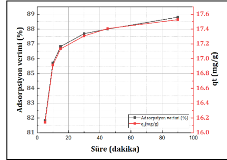
Şekil 6. Temas süresinin boya giderim verimine etkisi ( C_0=100 mg/L, 5g/L KST, pH 3, 25 °C, 200 rpm).
