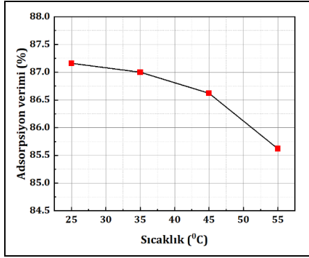
Şekil 7. Sıcaklığın boya giderim verimine etkisi ( C_0=100 mg/L, 5g/L KST, pH 3, 10 dk, 200 rpm).
