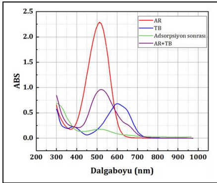
Şekil 8. Çözeltide bulunan farklı boyaların adsorpsiyona etkisi.
