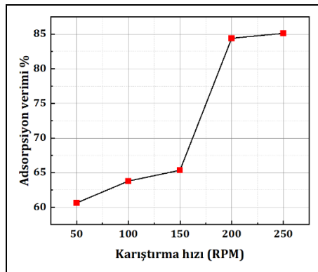
Şekil 5. Karıştırma hızının boya giderim verimine etkisi ( C_0=100 mg/L, 5g/L KST, pH 3, 25 °C, 60 dk.).
