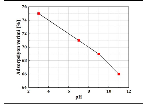
Şekil 3. Çözelti pH'ının boya giderim verimine etkisi ( C_0=100 mg/L, 10g/L KST, 25 °C, 60 dk, 150 rpm).
