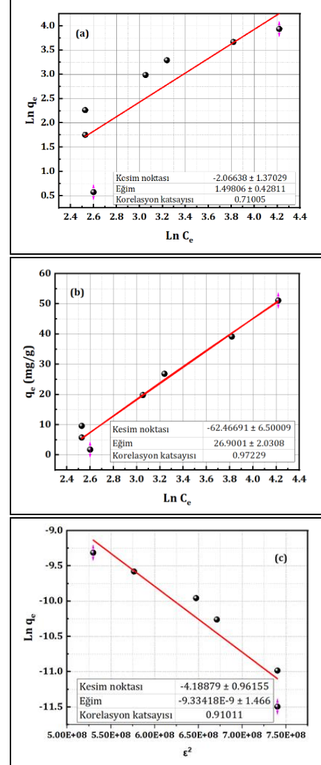
Şekil 9. Adsorpsiyon izoterm grafikleri a. Freundlich, b. Temkin, c. Dubinin Radushkevich.
