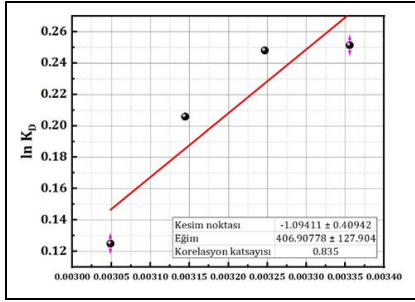
Şekil 11. KST üzerinde TB adsorpsiyona ait doğrusallaştırılmış Van't Hoff grafiği.
