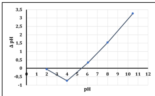
Şekil 2. pH drift yöntemi ile KST'nin pH_{pzc} tayini.
