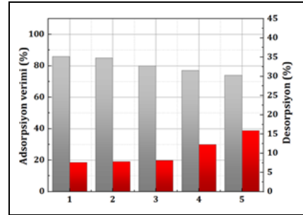
Şekil 12. KST'nin adsorpsiyon-desorpsiyon grafiği.
