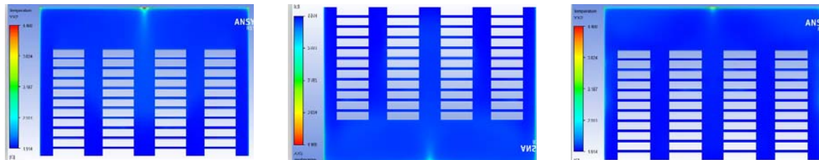
Şekil 13. Senaryo 1, 2 ve 3 için Z yönünde YX2 düzlemi için sıcaklık dağılımları
