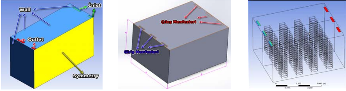
Şekil 5. Dış sınır şartları, katı model üzerinde giriş ve çıkış menfezleri ve depo kasa yerleşimi
