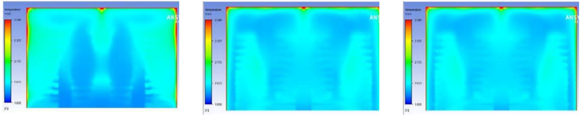
Şekil 16. Senaryo 1, 2 ve 3 için Z yönünde YX5 düzlemi için sıcaklık dağılımları
